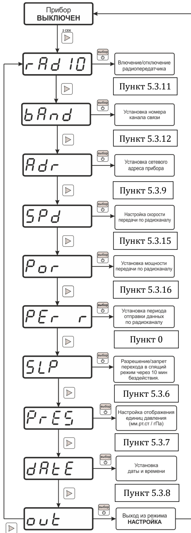
Рисунок 5.8 – Схема режима НАСТРОЙКА ИВТМ-7 М 4(-Д)
