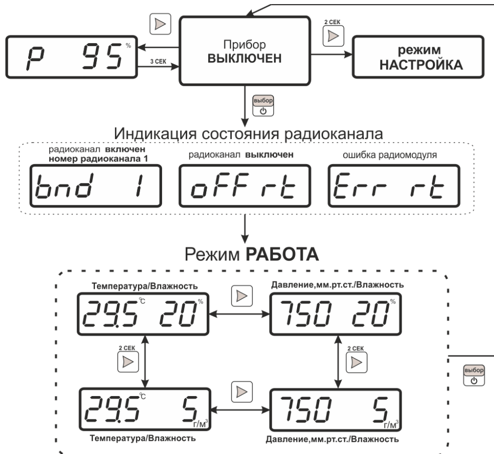
Рисунок 5.3 – Режим РАБОТА ИВТМ-7 М 4(-Д)
