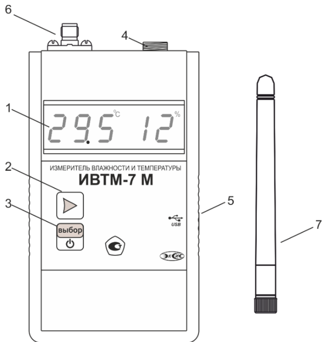
Рисунок 3.4 – Внешний вид измерительного блока ИВТМ-7 М 4(-Д)
