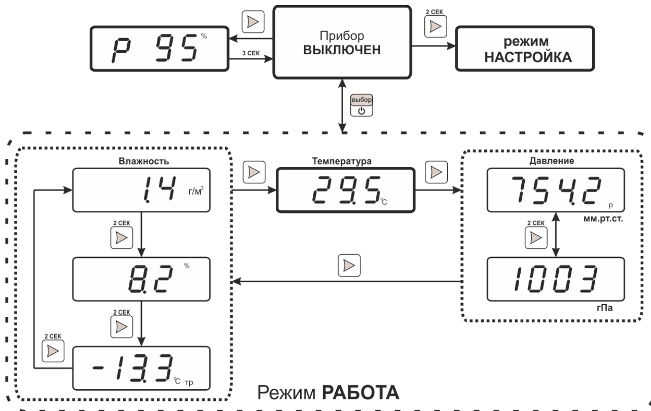
Рисунок 5.1 – Режим РАБОТА ИВТМ-7 М 1(-Д)
