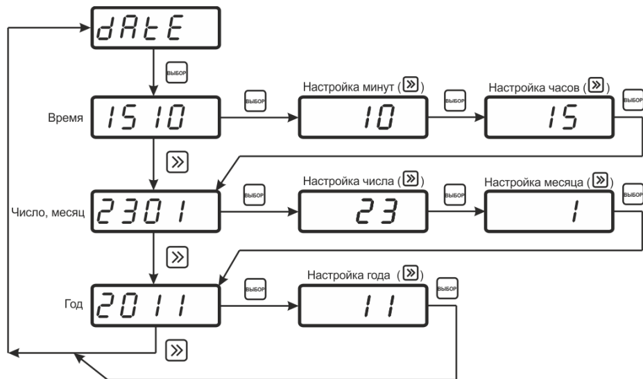
Рисунок 5.13 – Установка даты и времени
