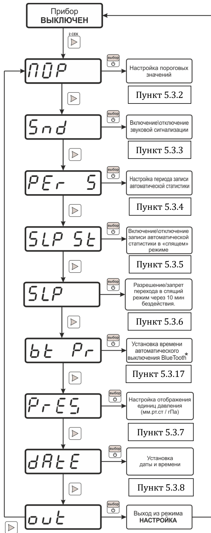
Рисунок 5.10 – Схема режима НАСТРОЙКА ИВТМ-7 М 7(-Д)
