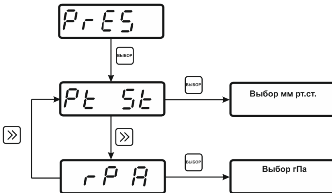
Рисунок 5.12 – Установка единиц отображения давления
