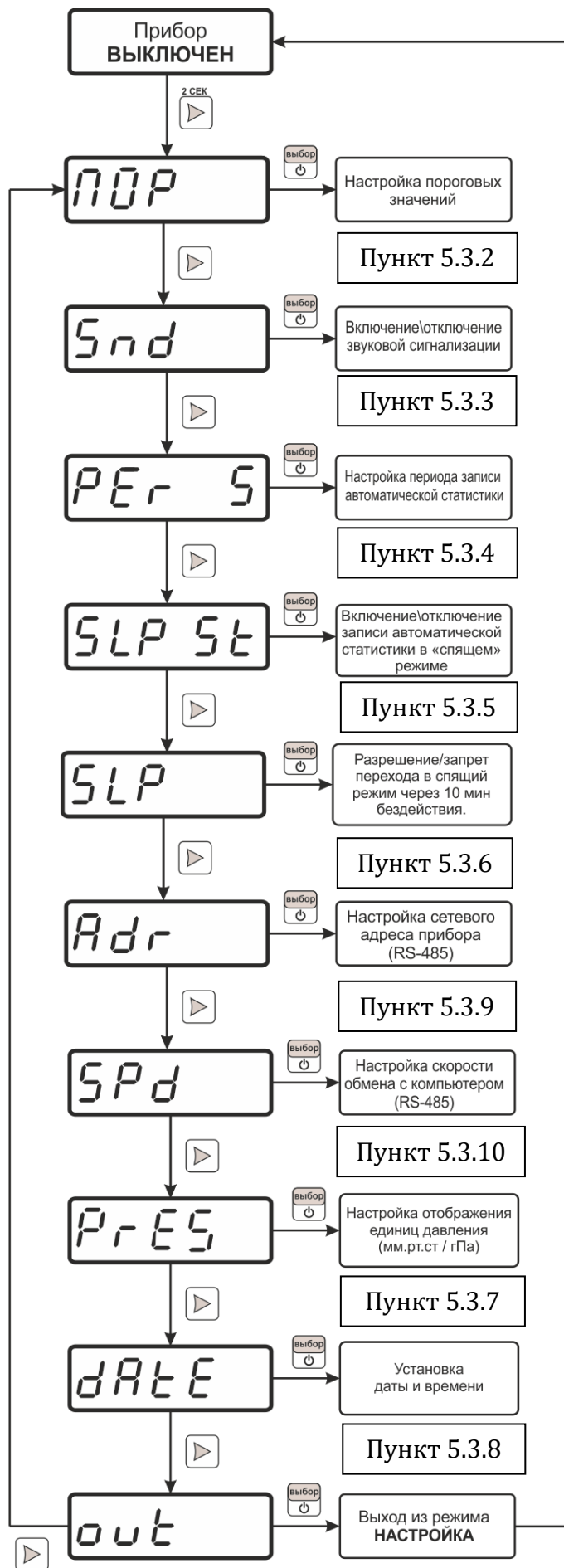
Рисунок 5.7 – Схема режима НАСТРОЙКА ИВТМ-7 М 3(-Д)
