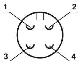
Разъем PC4 (вилка) со стороны монтажа
