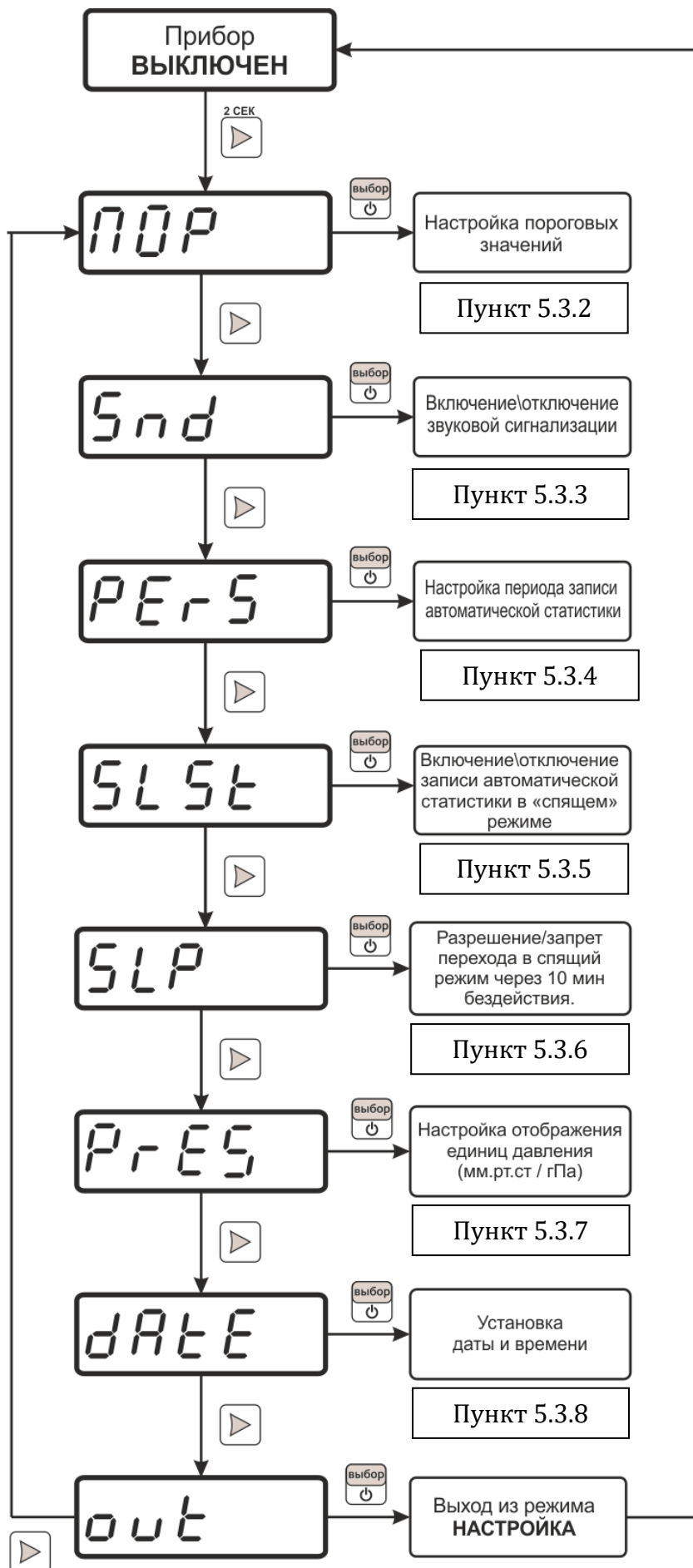
Рисунок 5.5 – Схема режима НАСТРОЙКА ИВТМ-7 М 1
