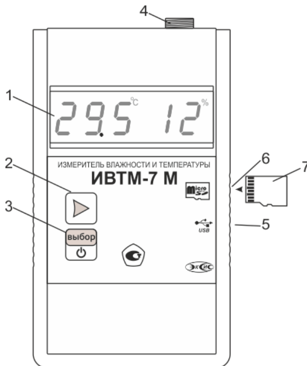
Рисунок 3.6 – Внешний вид измерительного блока ИВТМ-7 М 6(-Д)
