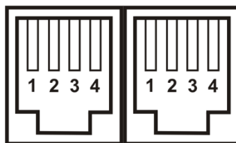
Рисунок 3.3 – Распиновка разъёмов подключения к сети RS-485
