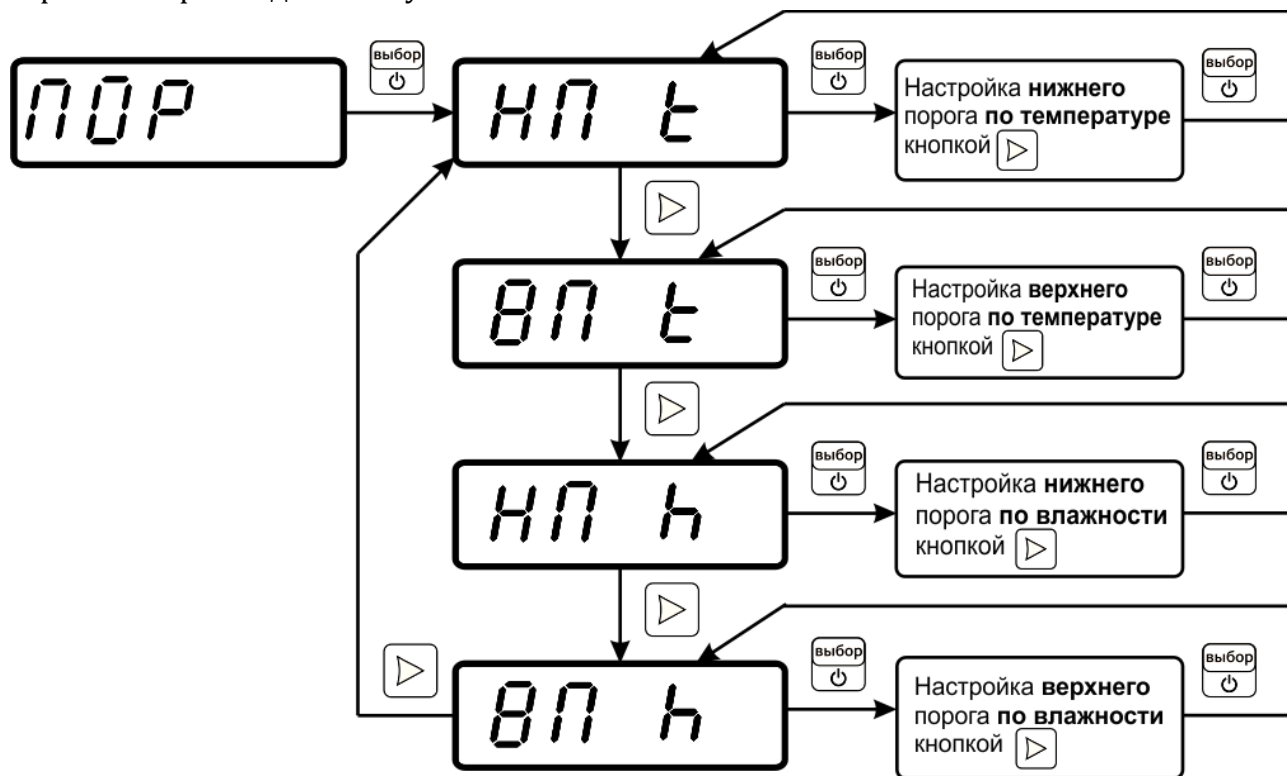
Рисунок 5.11 – Установка пороговых значений
