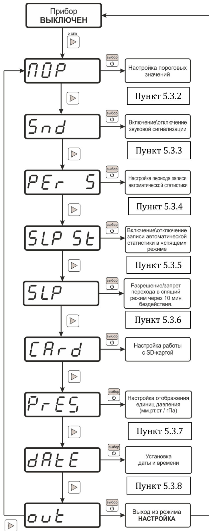
Рисунок 5.9 – Схема режима НАСТРОЙКА ИВТМ-7 М 6(-Д)
