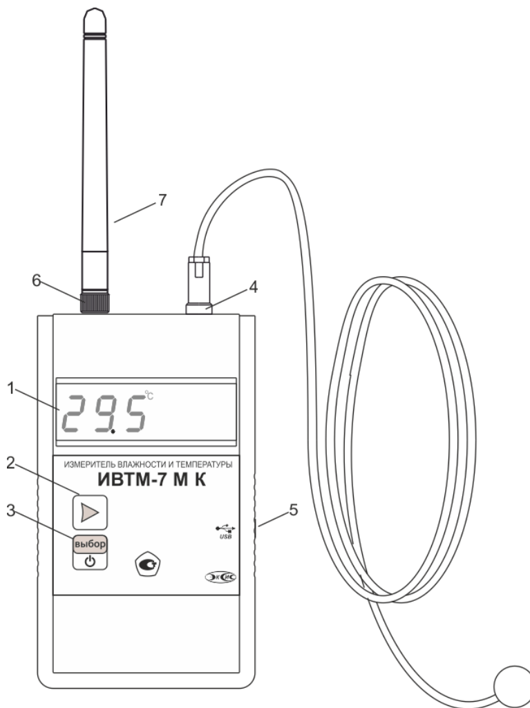
Рисунок 3.5а – Внешний вид измерительного блока ИВТМ-7 М 4 с зондом «монетой»
