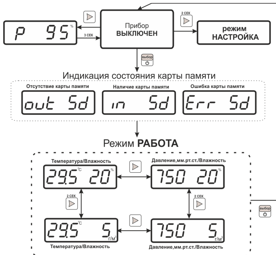
Рисунок 5.4 – Режим РАБОТА ИВТМ-7 М 6(-Д)
