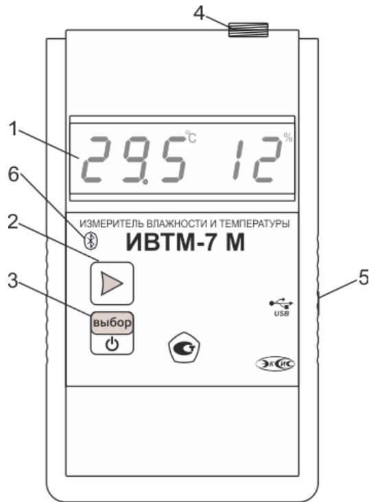
Рисунок 3.7 – Внешний вид измерительного блока ИВТМ-7 М 7(-Д)
