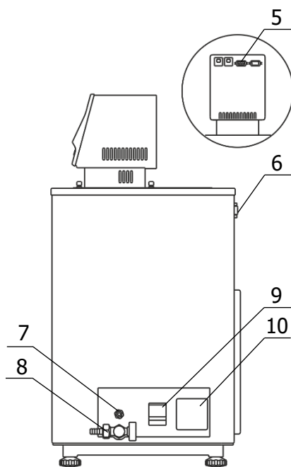
Рисунок 3 — Боковая панель термостата
