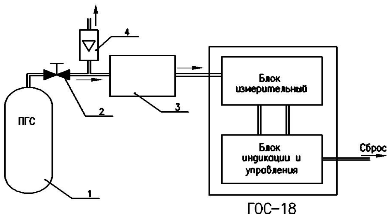
Рис. 4 – Схема подключения анализатора при проверке нуля измерительного канала:
