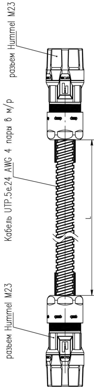
Схема электрическая соединений (Кабель Светоприемника)
