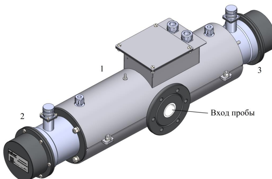
Рис. 2 Блок измерительный
