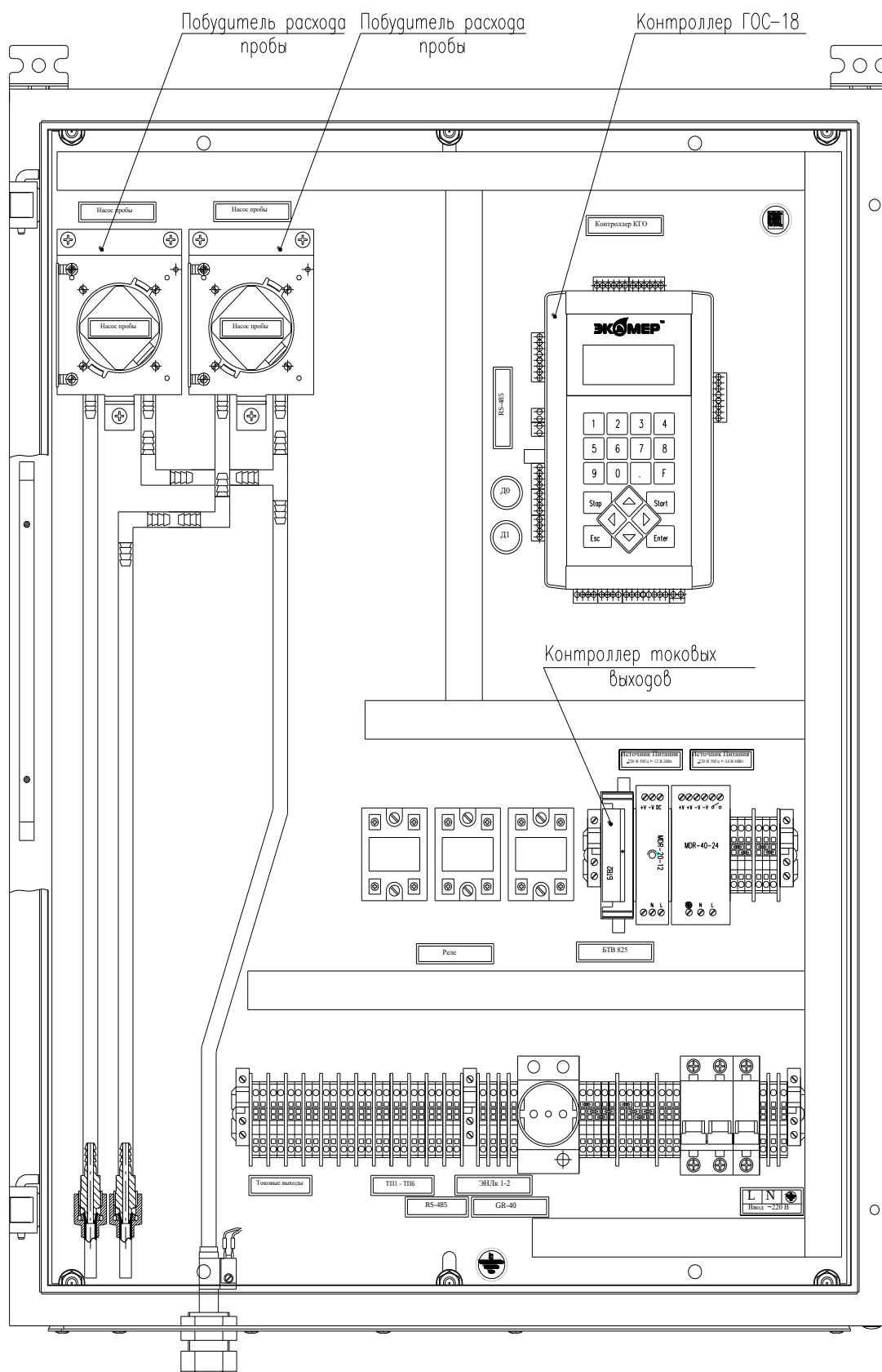
Рис. 1 Блок индикации и управления
