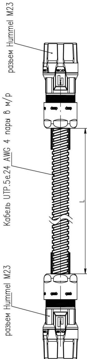
Схема электрическая соединений (Кабель Светоизлучателя)
