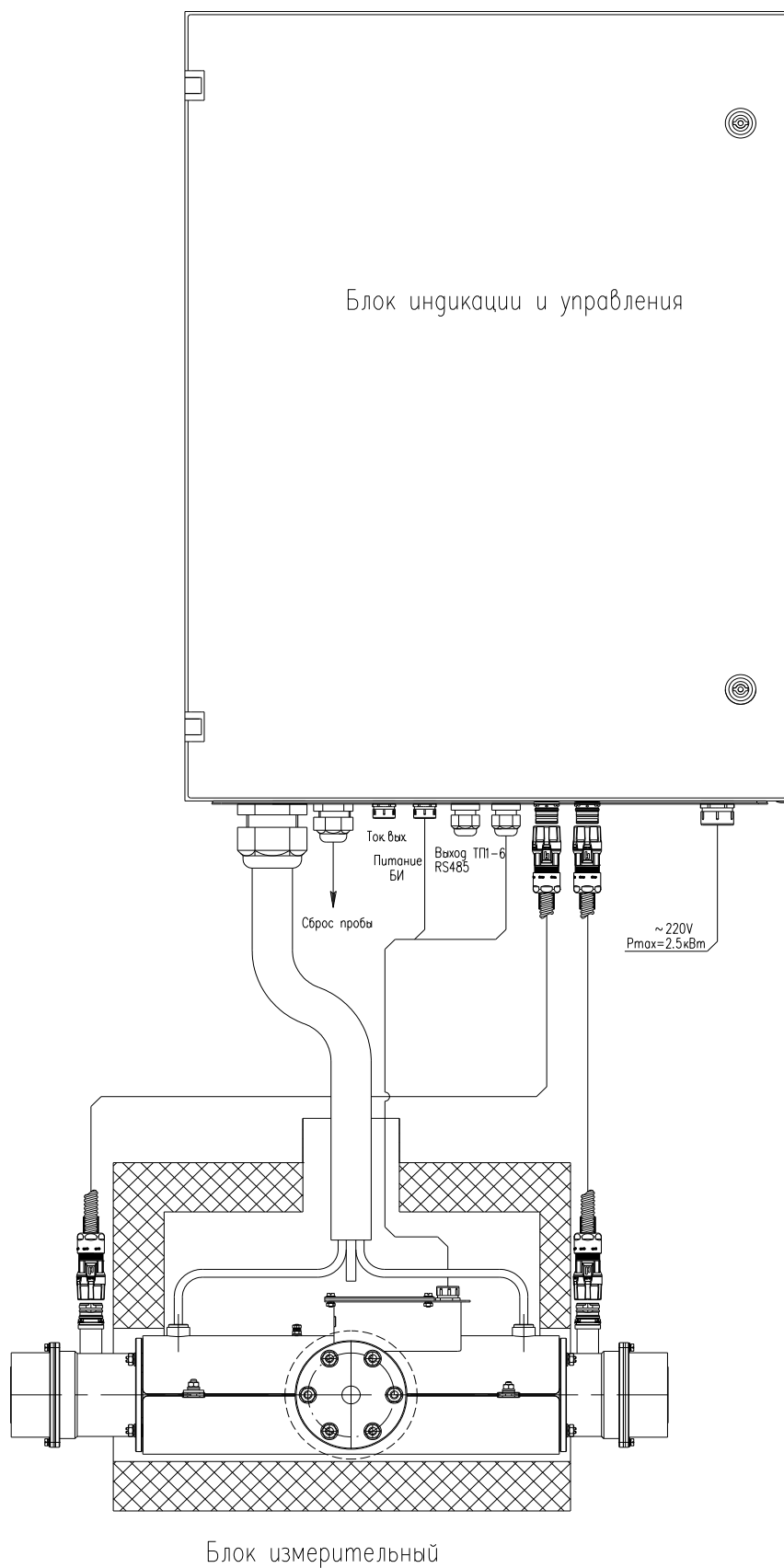
Рис. П.1 – Монтажный эскиз ГОС-18
